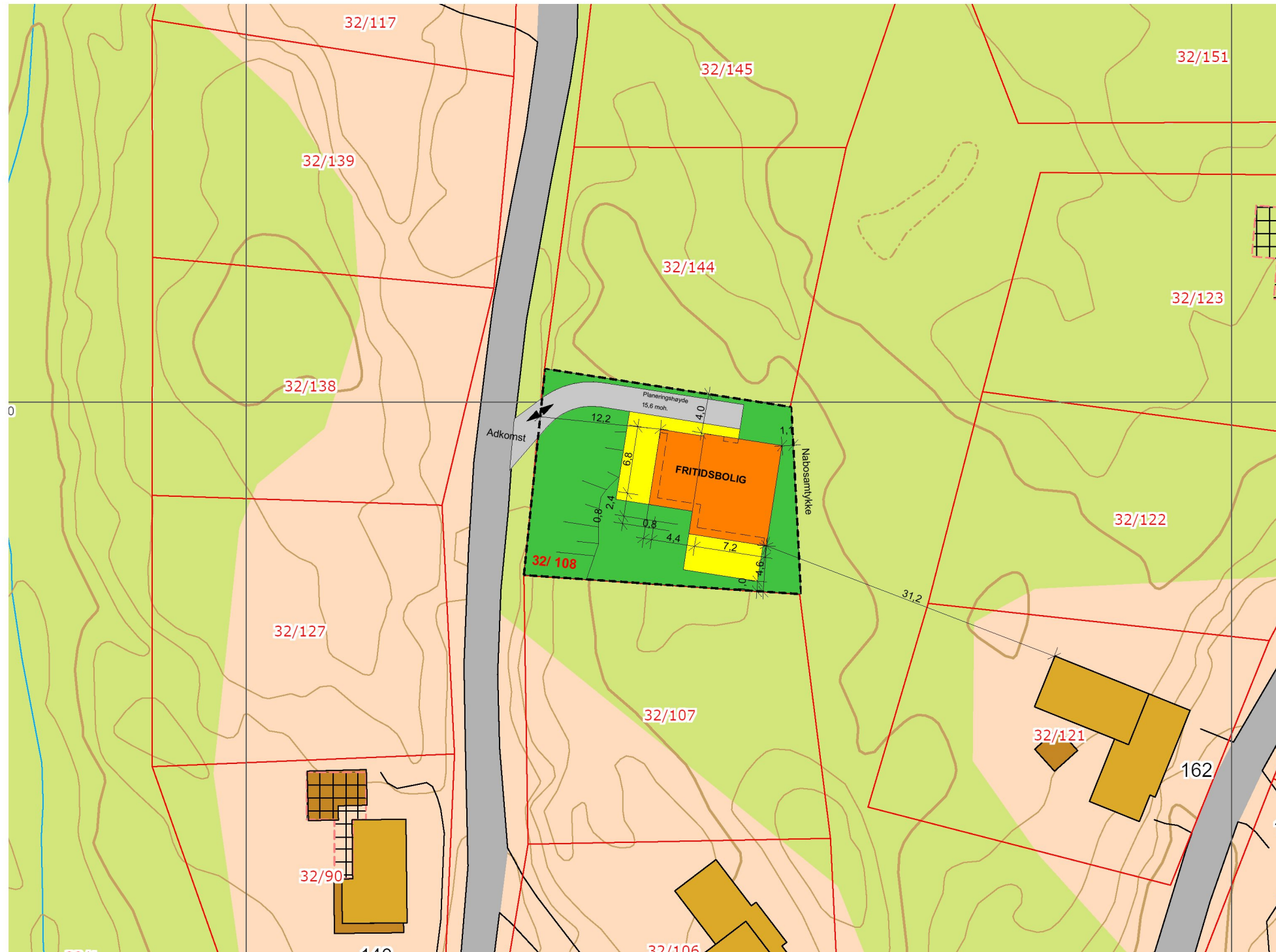
1:500 Situasjonsplan
